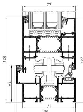
przekrój dolny drzwi z uszczelnieniem przyrywkowym
